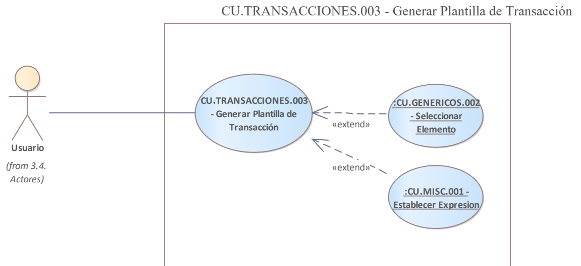
Figure 54: CU.TRANSACCIONES.003 - Generar Plantilla de Transacción
