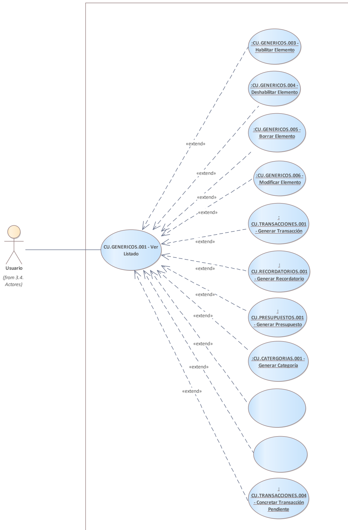
Figure 45: CU.GENERICOS.001 - Ver Listado
